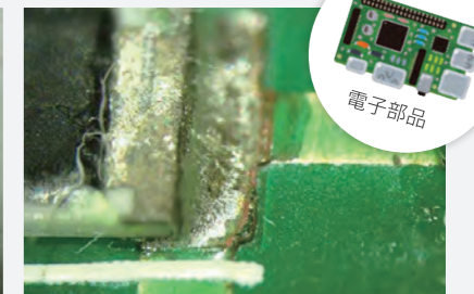
▲電子部品のパターンも腐食させてしまいます
